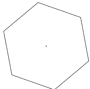
regelmässiges Sechseck
