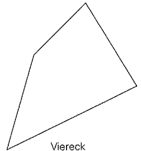
Viereck
