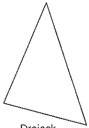
Dreieck
