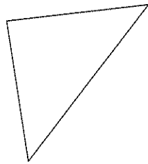
gleichschenkliges Dreieck
